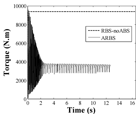
Fig. 15. Regenerative EM torque on icy road
